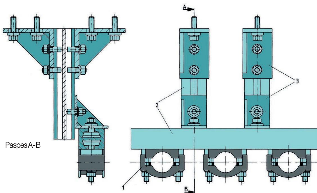
Крепление шины
